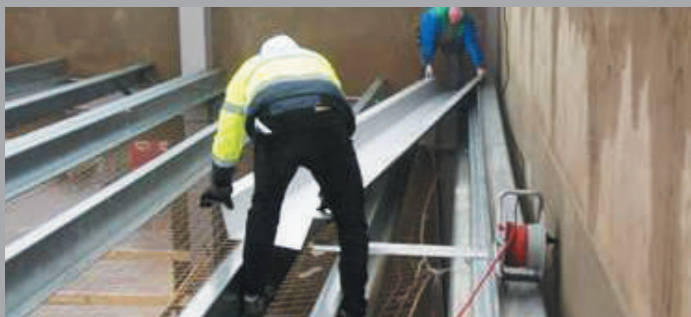
Установка нижнего желоба
